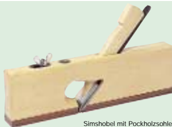
Simshobel mit Pockholzsohle
